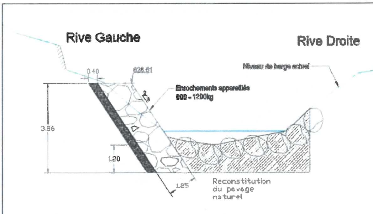
Enrochements appareillés/non-liasonnés
