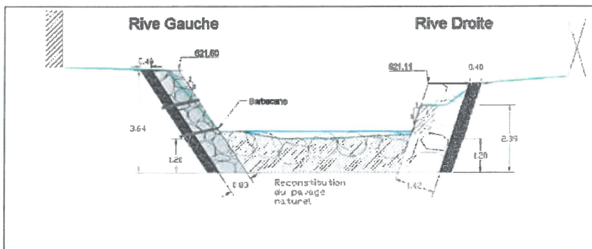
Enrochements appareillés/non-liaisonnés
