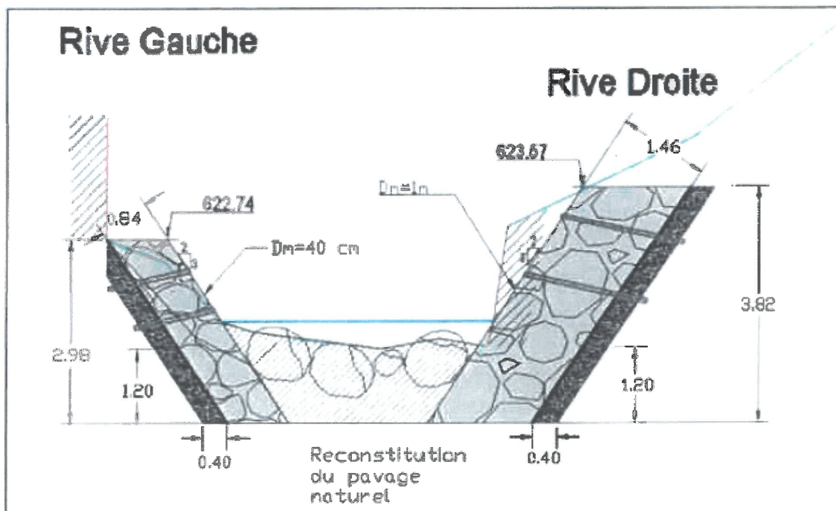
Enrochements bétonnés/liasonnés
