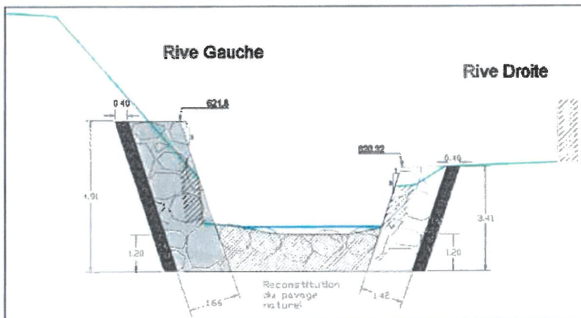
Enrochements bétonnés/liasonnés
