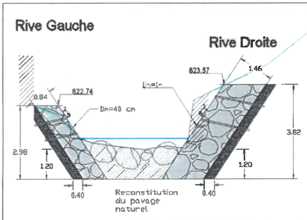
Enrochements liaisonnés/bétonnés
